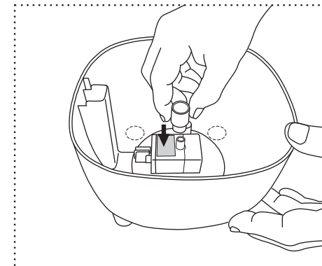
Stap 2 Bevestig de waterafvoerleiding aan de waterpomp.
