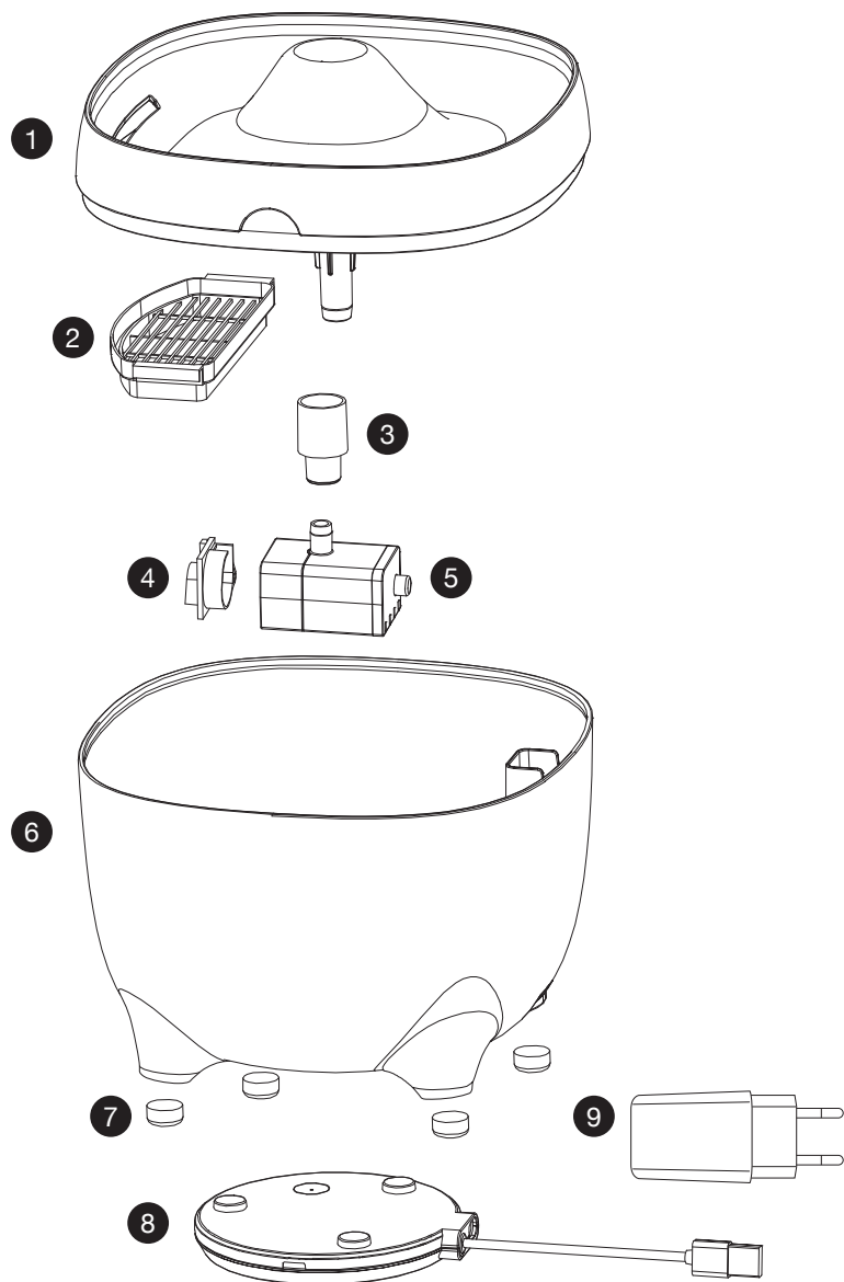
1. Wasserschale | 2. Filterhalter | 3. Wasserauslassrohr | 4. Pumpendeckel | 5. Kabellose wasserpumpe | 6. Wasserreservoir | 7. Anti-Rutsch-FüÙe | 8. Ladestation | 9. USB Transformator
