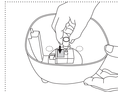
Schritt 2 Verbinden Sie das Wasserauslassrohr mit der Wasserpumpe
