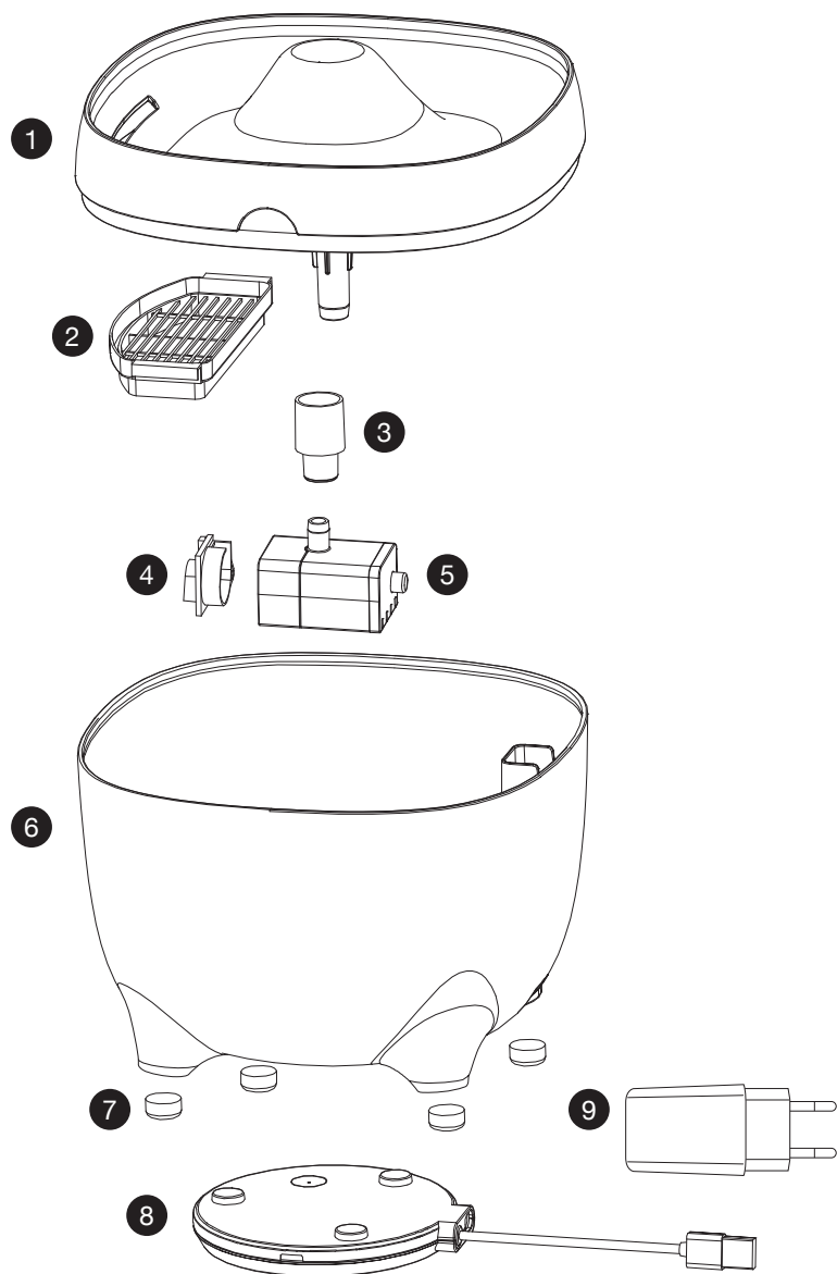
1. Waterdispenser | 2. Filter houder | 3. Waterafvoerleiding | 4. Pomp deksel | 5. Draadloze water pomp | 6. Water tank | 7. Anti slip voetjes | 8. Laadstation | 9. USB Adapter
